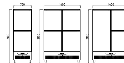
Versões meias portas com grupo inferior Half-door versions with lower group Versions demi-portes avec groupe inférieur
