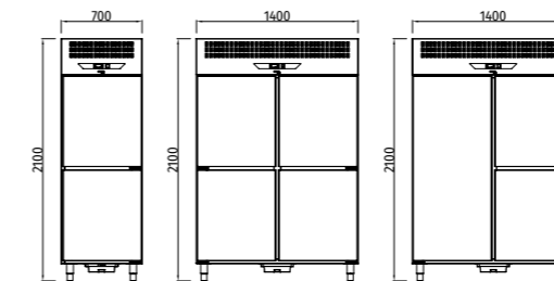
Versões meias portas com grupo superior Half-door versions with upper group Versions demi-portes avec groupe supérieur
