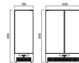
Versão vinhos com porta vidro Wine version with glass door Version vin avec porte vitrée
