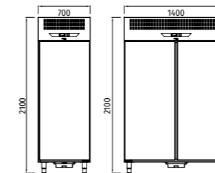
Versão porta inteira com grupo superior Full door version with upper group Version porte pleine avec groupe supérieur
