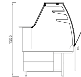
VCC VCC - Vidro côncavo / Concave glass / Vitrage concave
