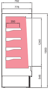
Com prateleiras aquecidas com grelhas With heated grid shelves Avec étagères chauffantes avec grilles
